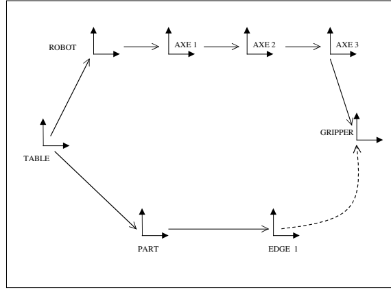
FIG. 2.6 – Graphe cinématique correspondant au problème d'inversion géométrique.
