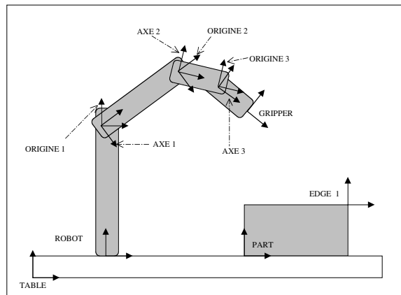
FIG. 2.9 – Exemple d'un problème simple d'inversion géométrique sous incertitudes géométriques. Ce problème consiste à ramener le point final du bras sur une arête d'un objet. Les longueurs des corps du bras, les zéros des articulations ainsi que les positions de la base ROBOT et de l'objet PART sont entachés d'incertitude.
